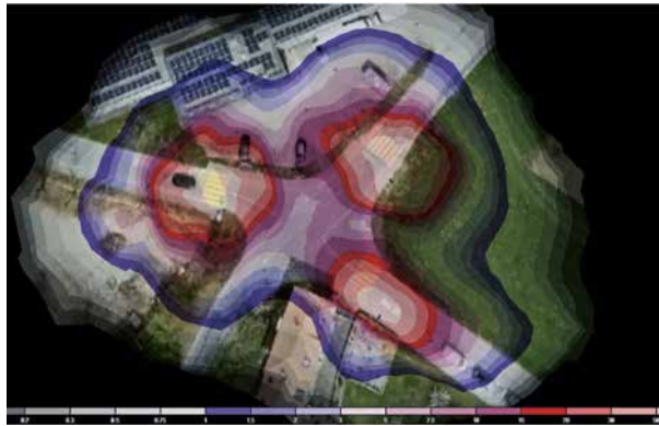
Exemple d'une étude photométrique du carrefour rue de la Gare/Trois-Rods.
