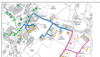
Le plan des travaux.
