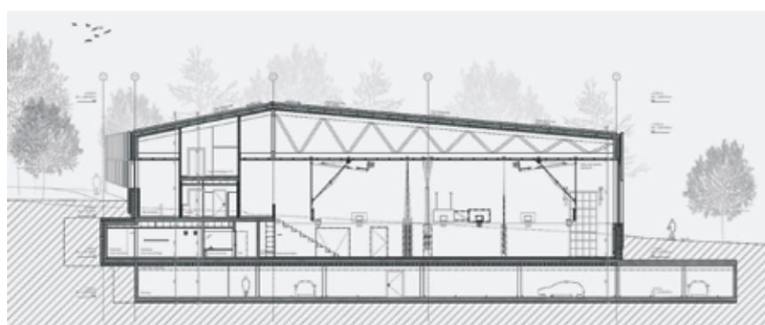
Coupe transversale de la future salle de gym. Le niveau inférieur avec les deux terrains de sport sera semi-enterréd avec le parking en-dessous.
